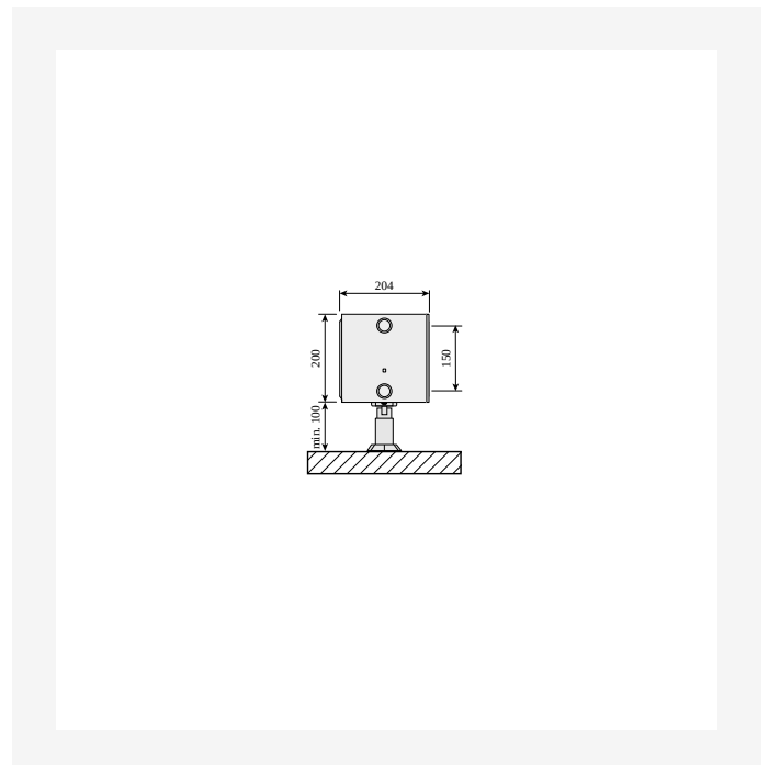
DimensionalDrawing - Plint P ja Plint R, tüüp 44, põrandakinnitustega, külgsaade
