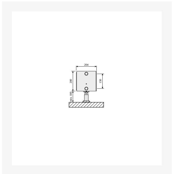
DimensionalDrawing - Plint P ja Plint R, tüüp 44, põrandakinnitustega, külgvaade
