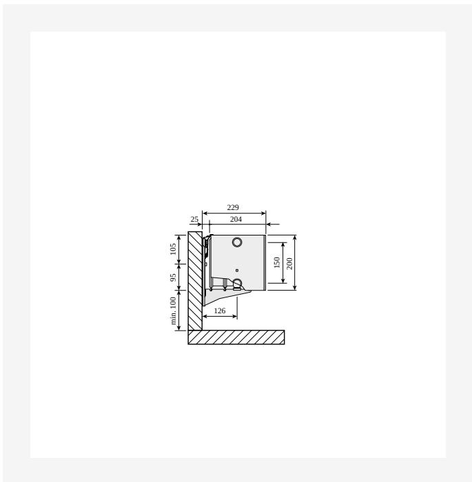
DimensionalDrawing - Plint P ja Plint R, tüüp 44, külgvaade Monclac seinakanduritega
