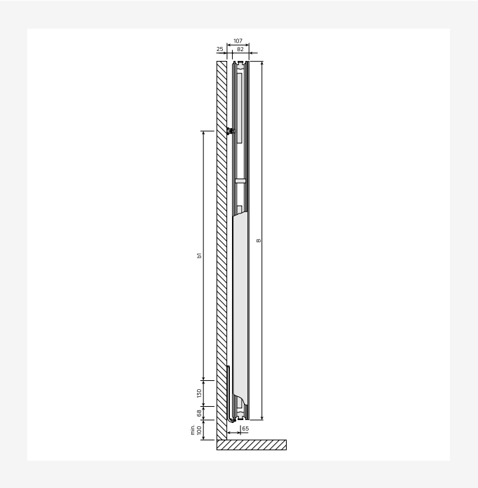
DimensionalDrawing - Kos V / Faro V, tüüp 21, külgvaade
