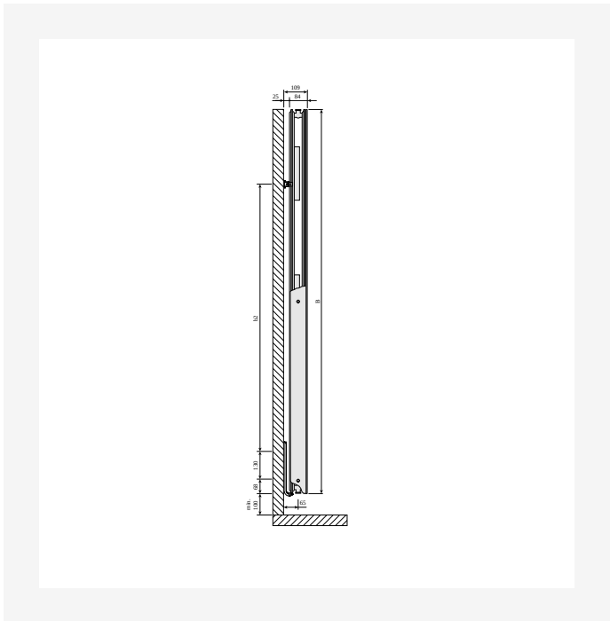
DimensionalDrawing - Kos V ja Faro V, tüüp 21, külgvaade
