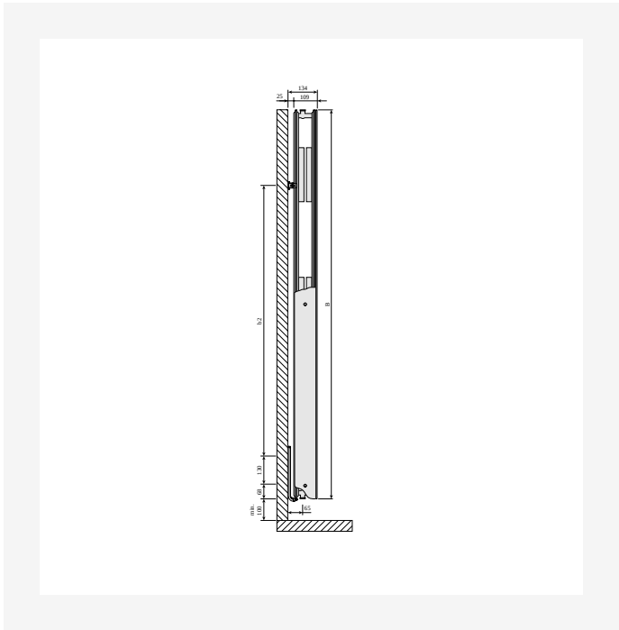
DimensionalDrawing - Kos V ja Faro V, tüüp 22, külgvaade
