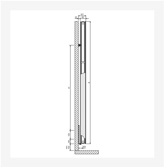
DimensionalDrawing - Kos V / Faro V, tüüp 20, külgvaade
