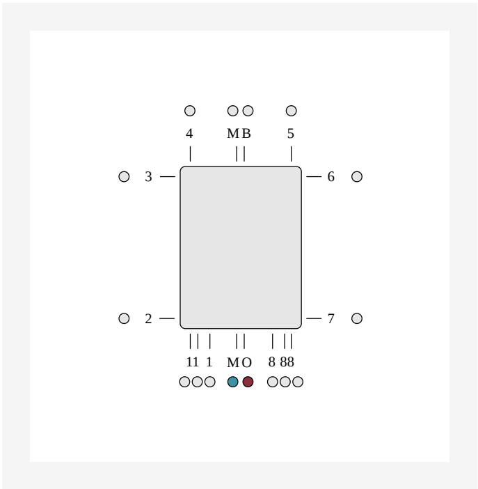
DimensionalDrawing - ETIM OM, vertikaalne keskühendus
