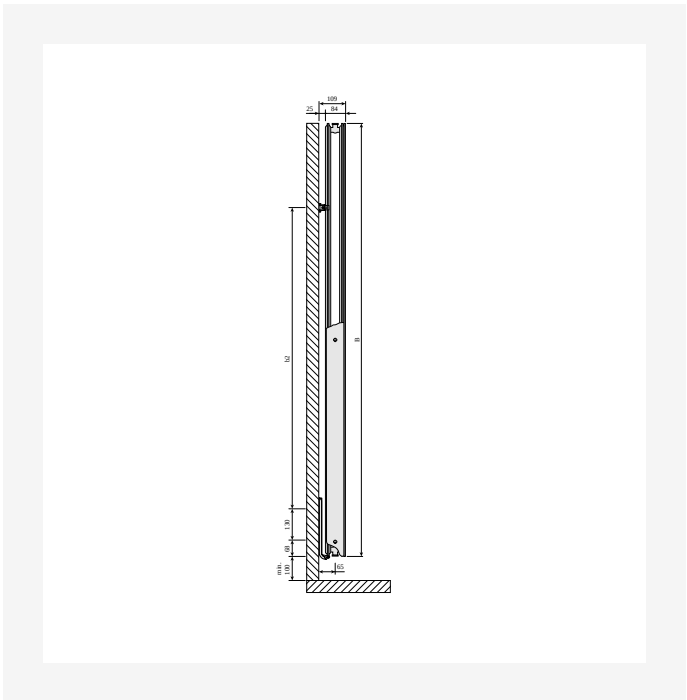
DimensionalDrawing - Kos V ja Faro V, tüüp 20, külgvaade
