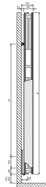
DimensionalDrawing - Kos V / Faro V, tüüp 22, külgsaade
