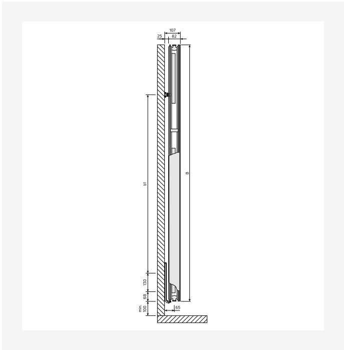
DimensionalDrawing - Kos V / Faro V, tüüp 21, külgvaade
