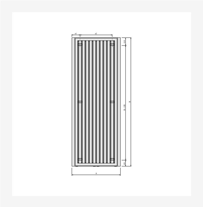
DimensionalDrawing - Paros V, bagfra
